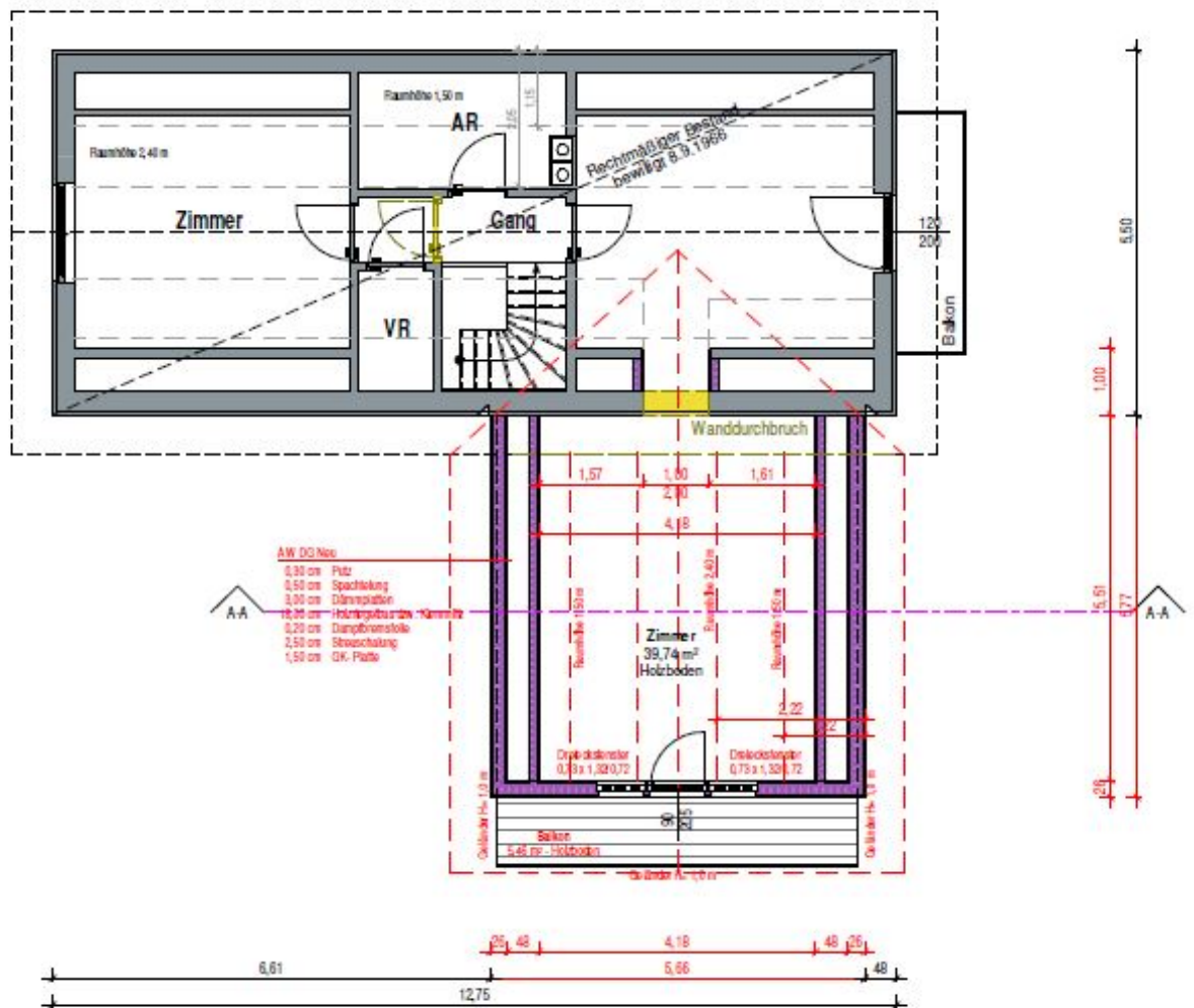
GRUNDRISS DACHGESCHOSS M 1:100
