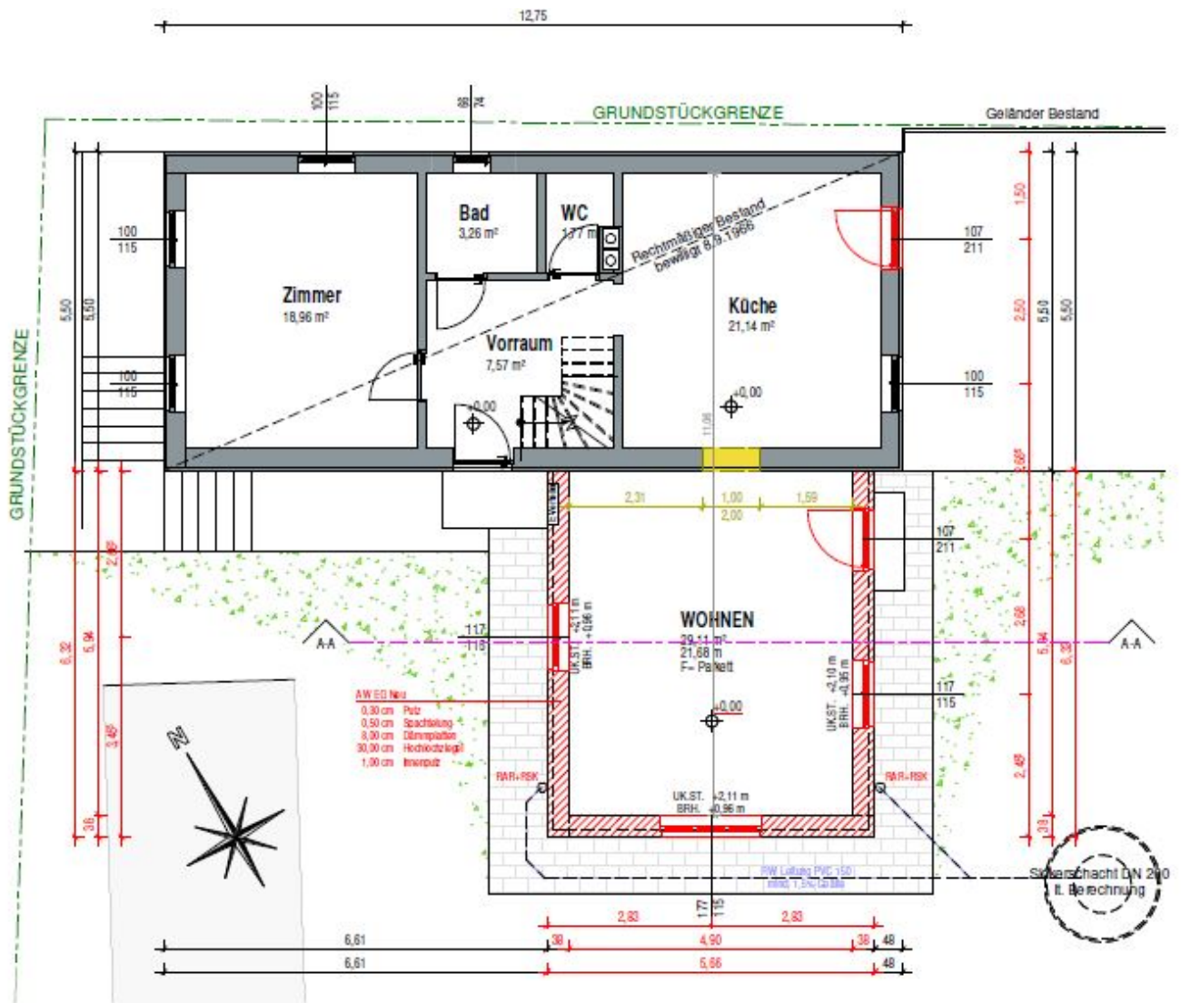
GRUNDRISS ERDGESCHOSS M 1:100
